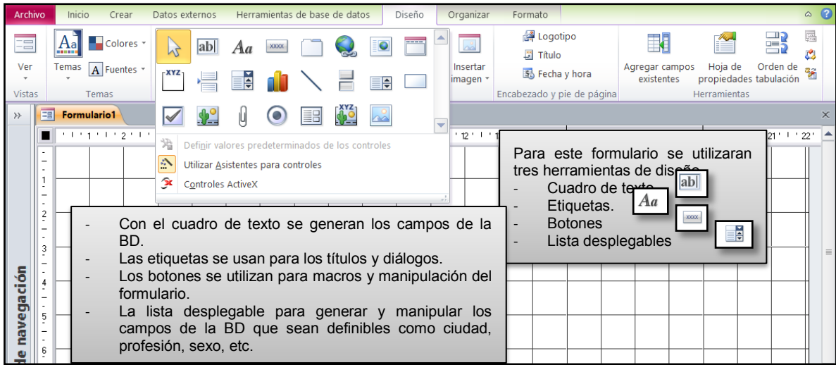
Figura 43. Formulario en vista de diseño
