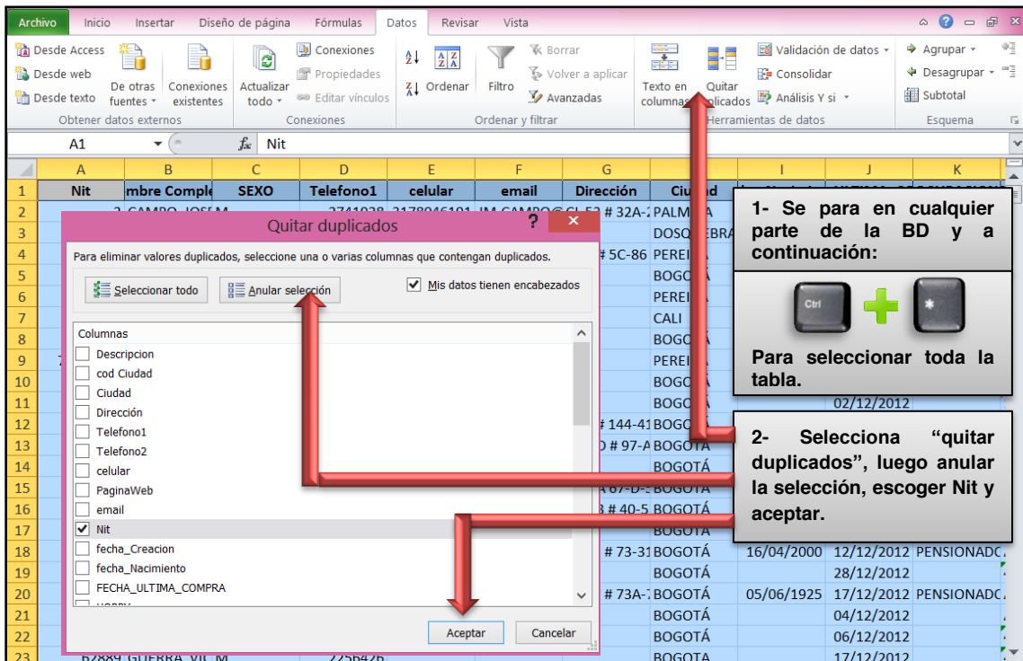
Figura 22. Eliminar los registros repetidos
