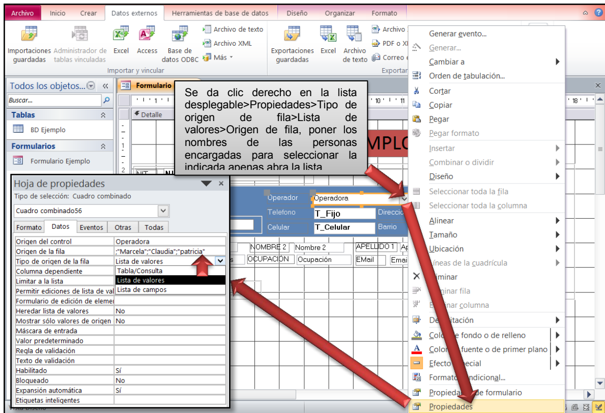
Figura 47. Dar valores en la lista desplegable directamente
