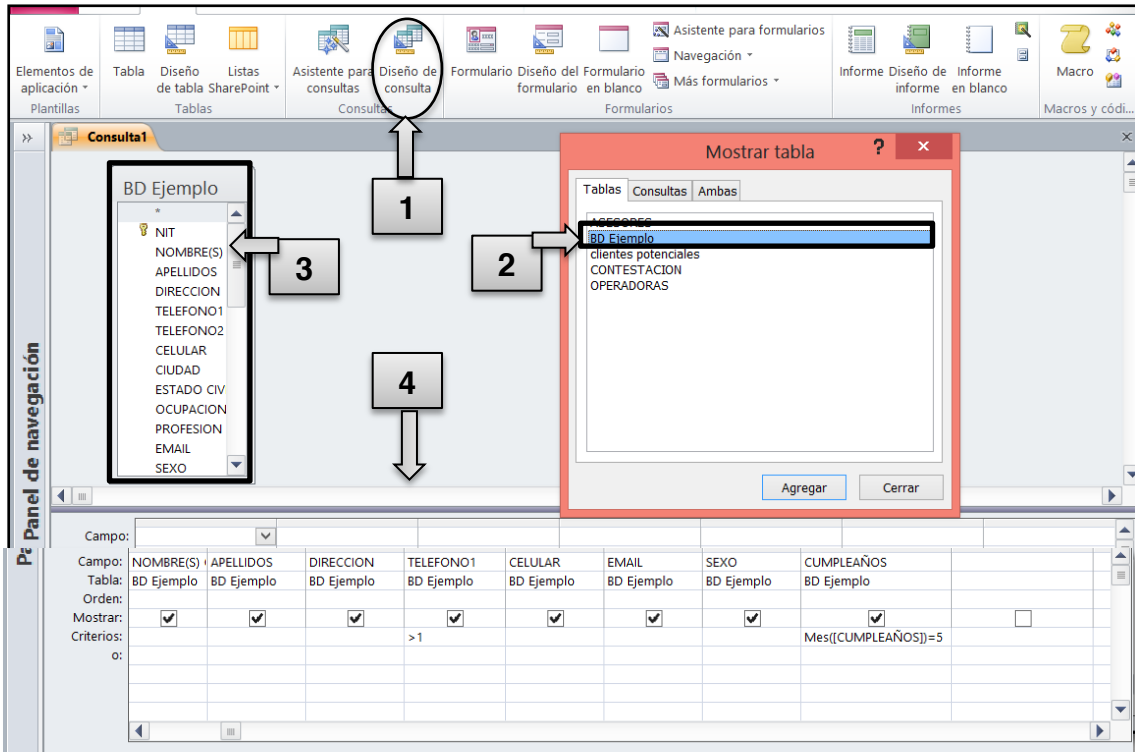
Figura 15. Consulta vista de diseño cumpleaños (teléfonos fijos)
