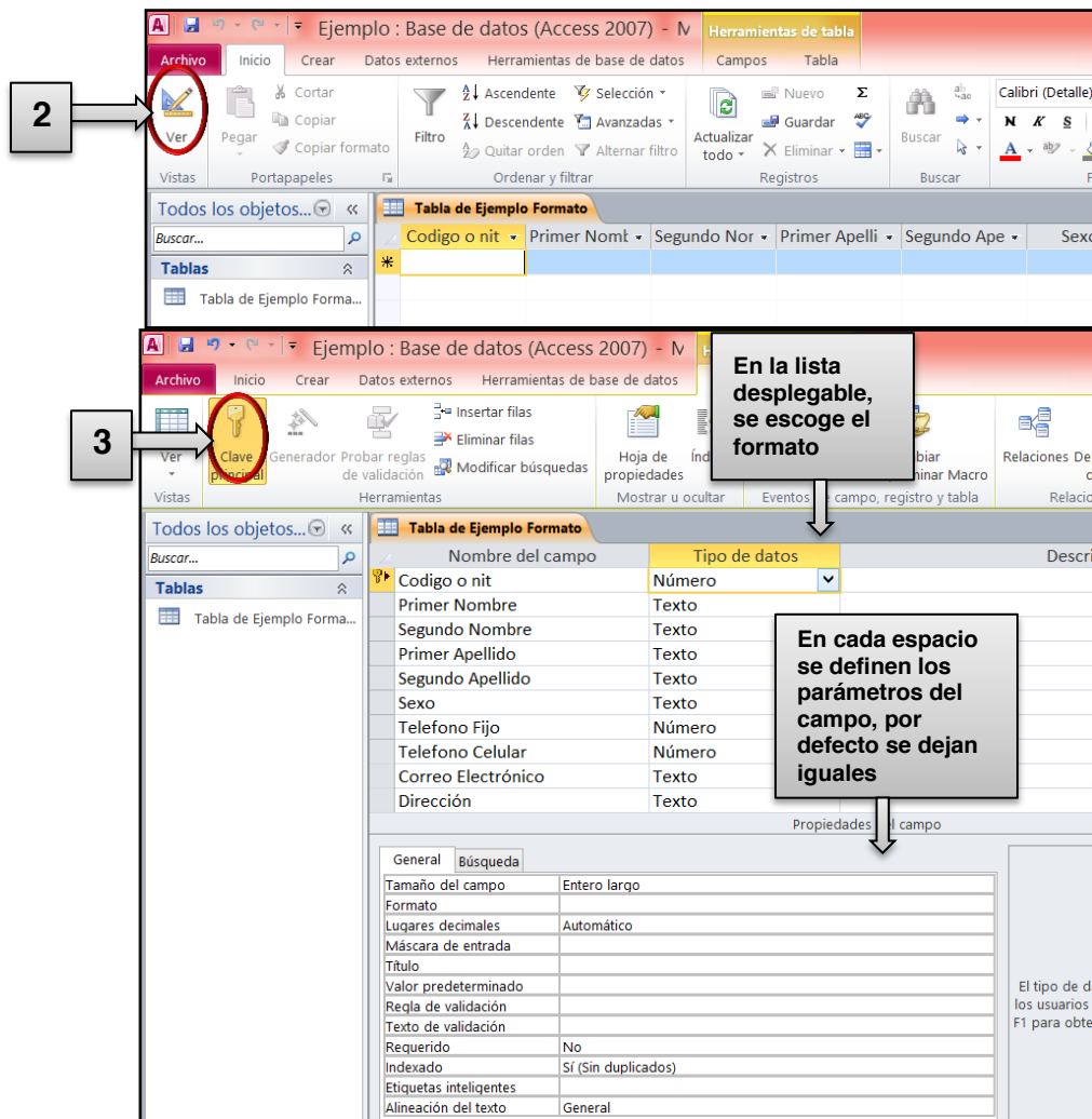
Figura 6. Formatear texto en Access
